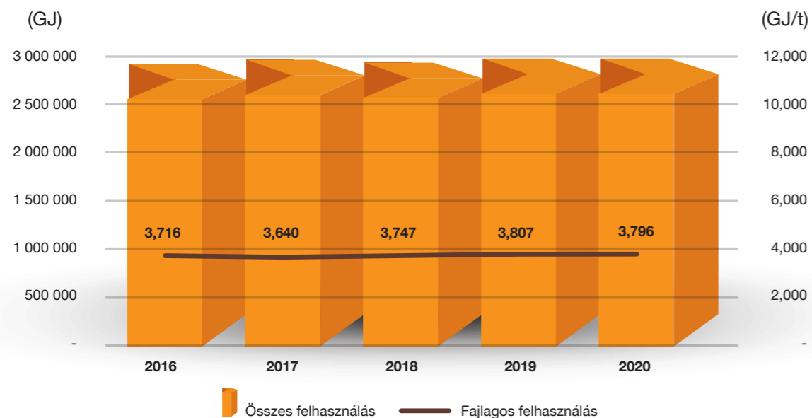
A papírgyártás összes hőenergia felhasználásának alakulása
